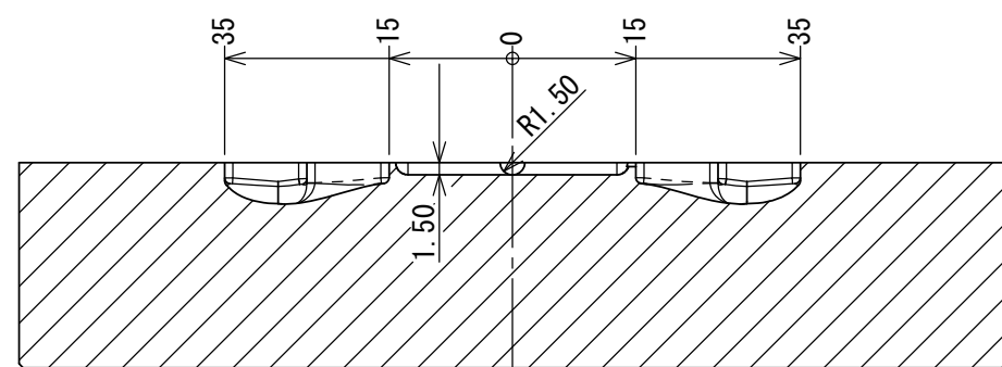
断面図 B-B
